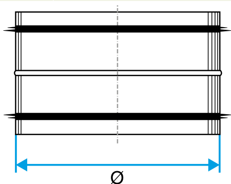
Schéma d'encombrement Raccord Mâle à joints
