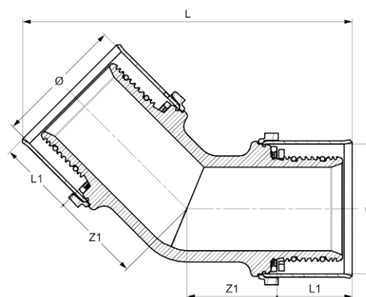
Vue en coupe avec cote
