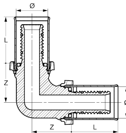
Vue en coupe avec cote
