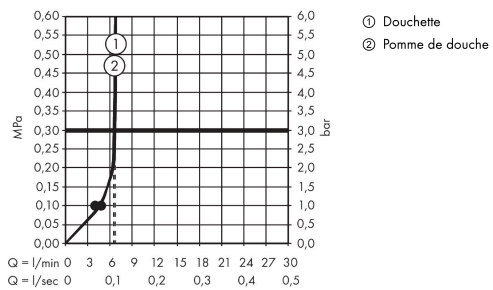
Schéma d'écoulement
