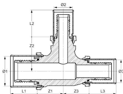
Vue en coupe avec cote
