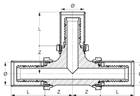
Vue en coupe avec cote
